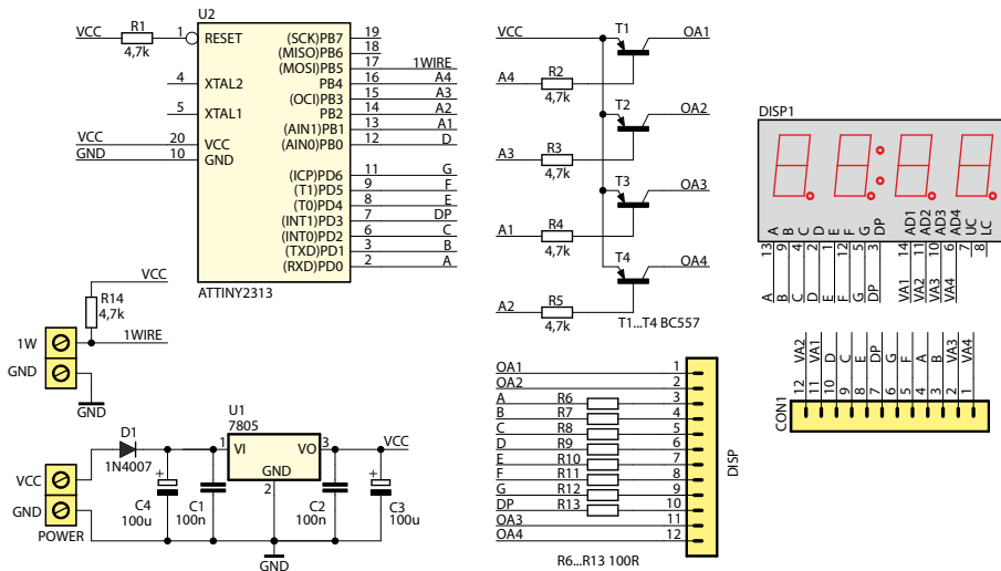
Rys. 3. Schemat ideowy
